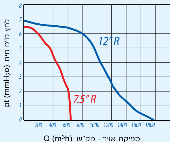
עקומת לחץ / ספיקת אוויר
